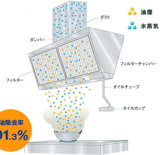
アルファフィルターII 油煙通過イメージ
